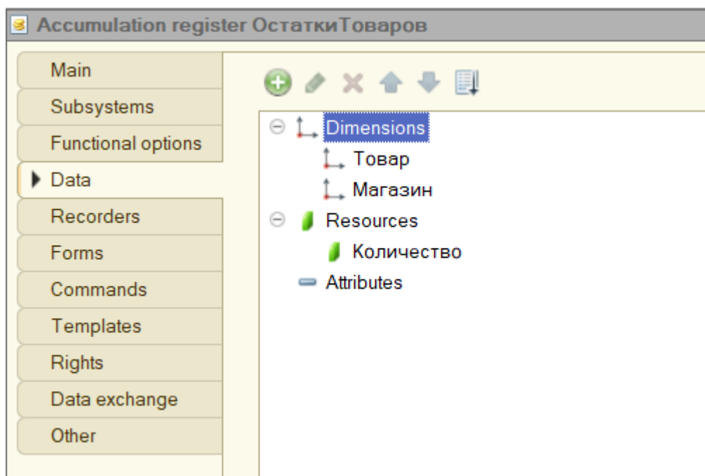
Рисунок 2.1.19 – Регистр накопления “ОстаткиТоваров”
