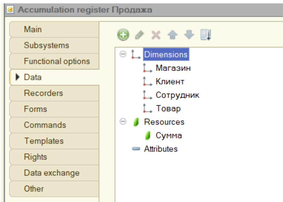
Рисунок 2.1.16 – Регистр накопления “Продажа”
