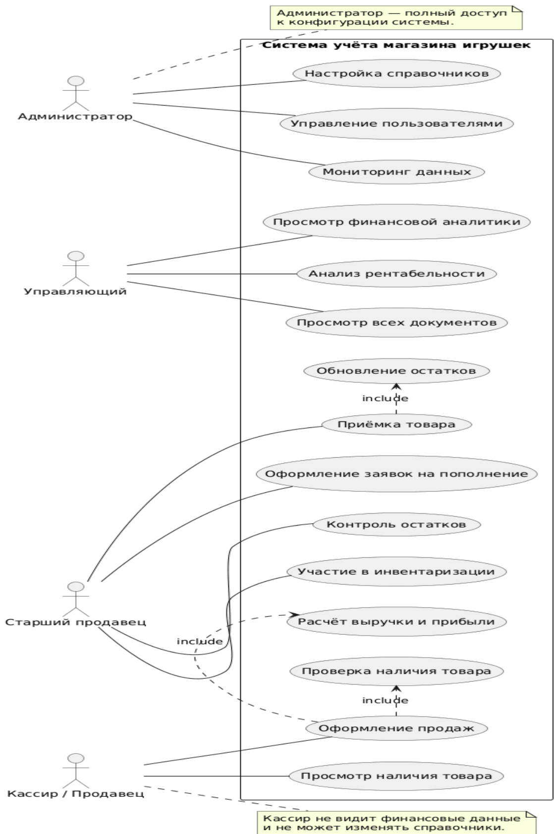
Рисунок 1.1 – Диаграмма вариантов использования системы
