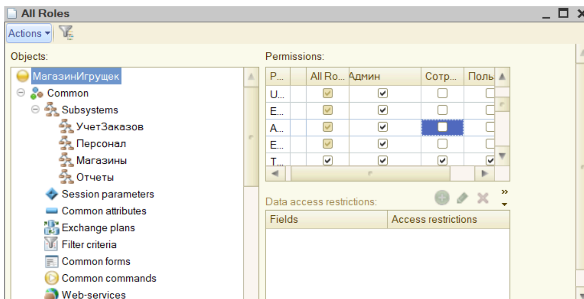
Рисунок 4.1 – Разграничение прав доступа по ролям пользователей
